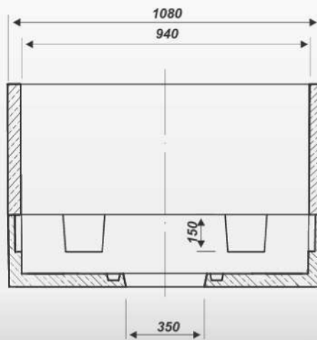
Przekrój podłużny
