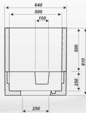
Przekrój poprzeczny
